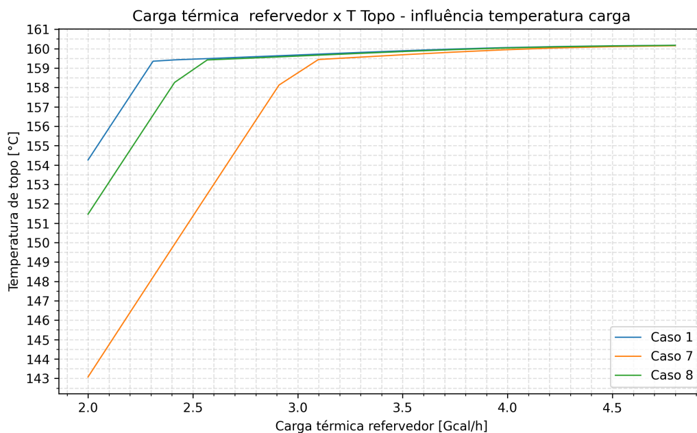
Figura 9: Carga térmica x temperatura do topo - Influência da temperatura da carga
